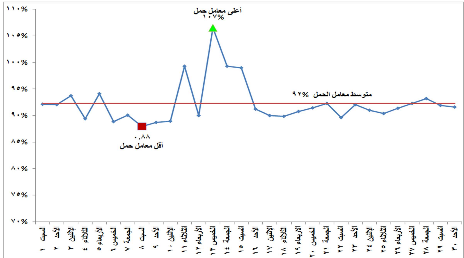
شكل (١٢) إجمالي معامل الحمل لوحدات الانتاج خلال شهر يونيو ٢٠١٩
