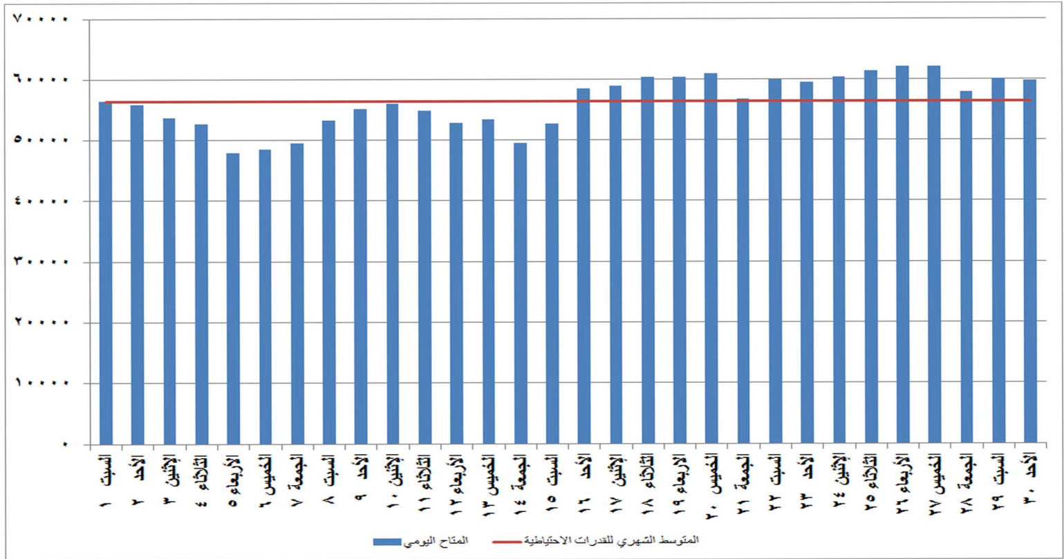
شكل (٢٧) القدرات المتاحة يوميا والمتوسط الشهري للقدرة الاحتياطية خلال شهر يونيو ٢٠١٩
