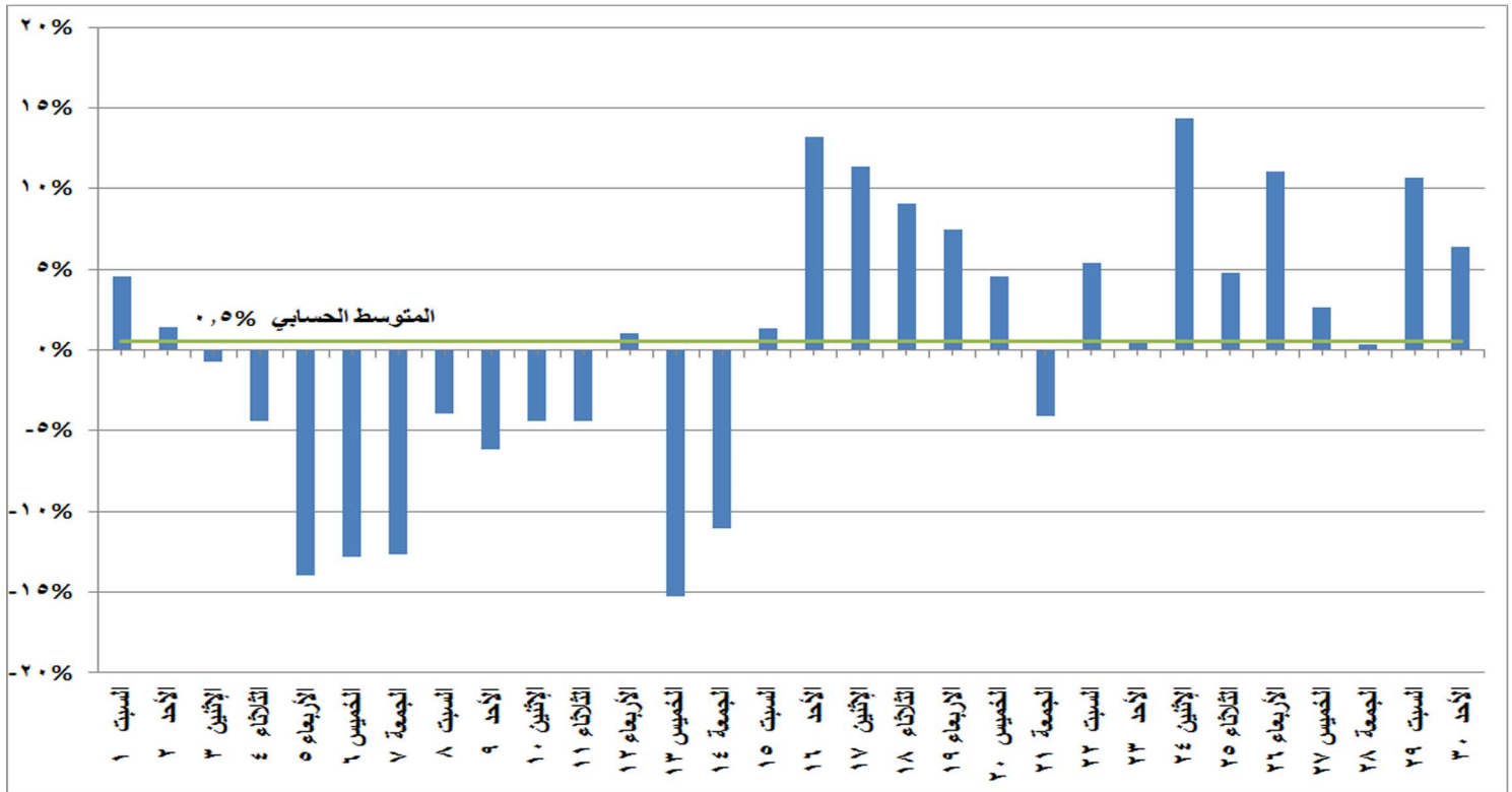
شكل (٩) النسب المئوية للتغير في الحمل الاقصى خلال شهر يونيو ٢٠١٩ مقارنة باليوم المماثل من العام الماضي
