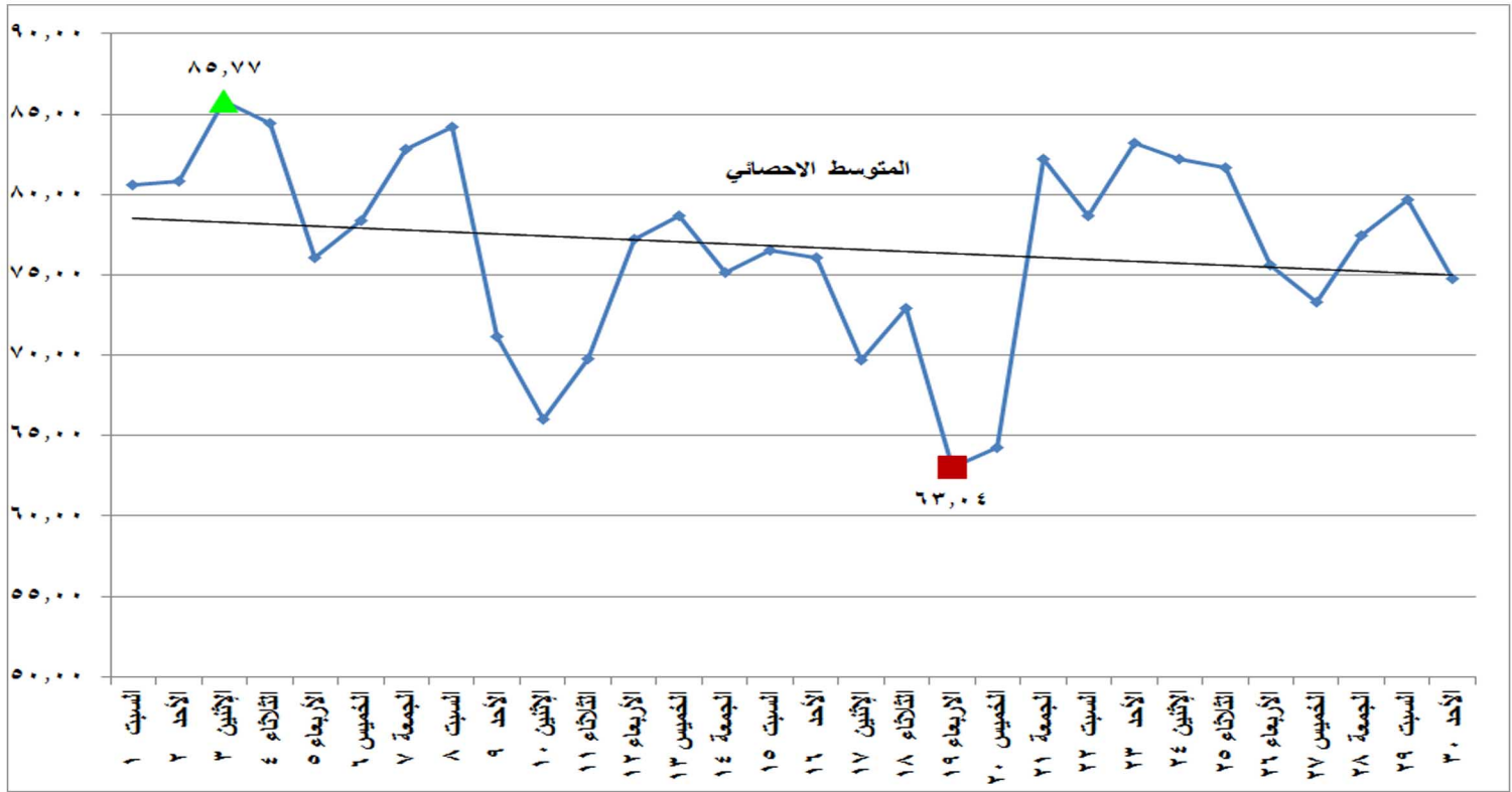
شكل (٢١) الطاقة الكهربائية المنتجة من المصادر غير الحرارية خلال شهر يونيو ٢٠١٩
