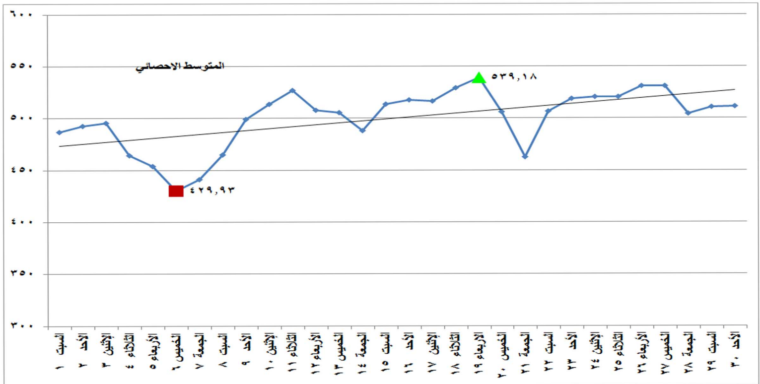
شكل (١٧) الطاقة الكهربائية المنتجة من الغاز الطبيعي خلال شهر يونيو ٢٠١٩
