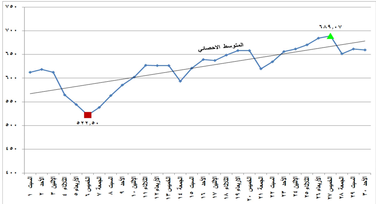
شكل (١٥) إجمالي الطاقة الكهربائية المنتجة من كل المصادر الأولية خلال شهر يونيو ٢٠١٩
