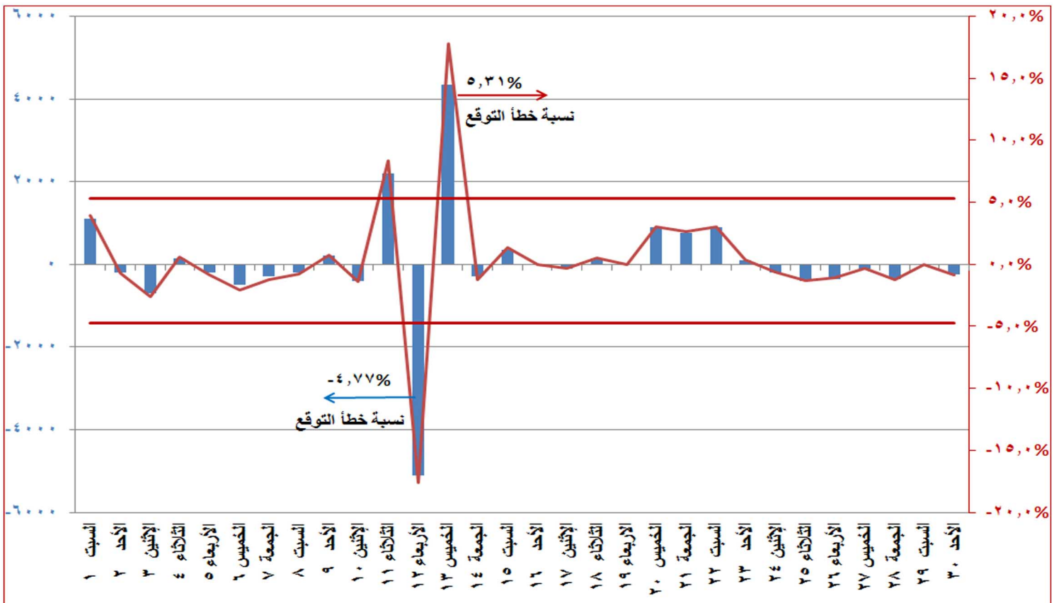
شكل (١٠) الفرق بين الحمل الأقصى المتوقع والمسجل فعليا ونسبة الفرق إلى الحمل المسجل فعليا خلال شهر يونيو ٢٠١٩
