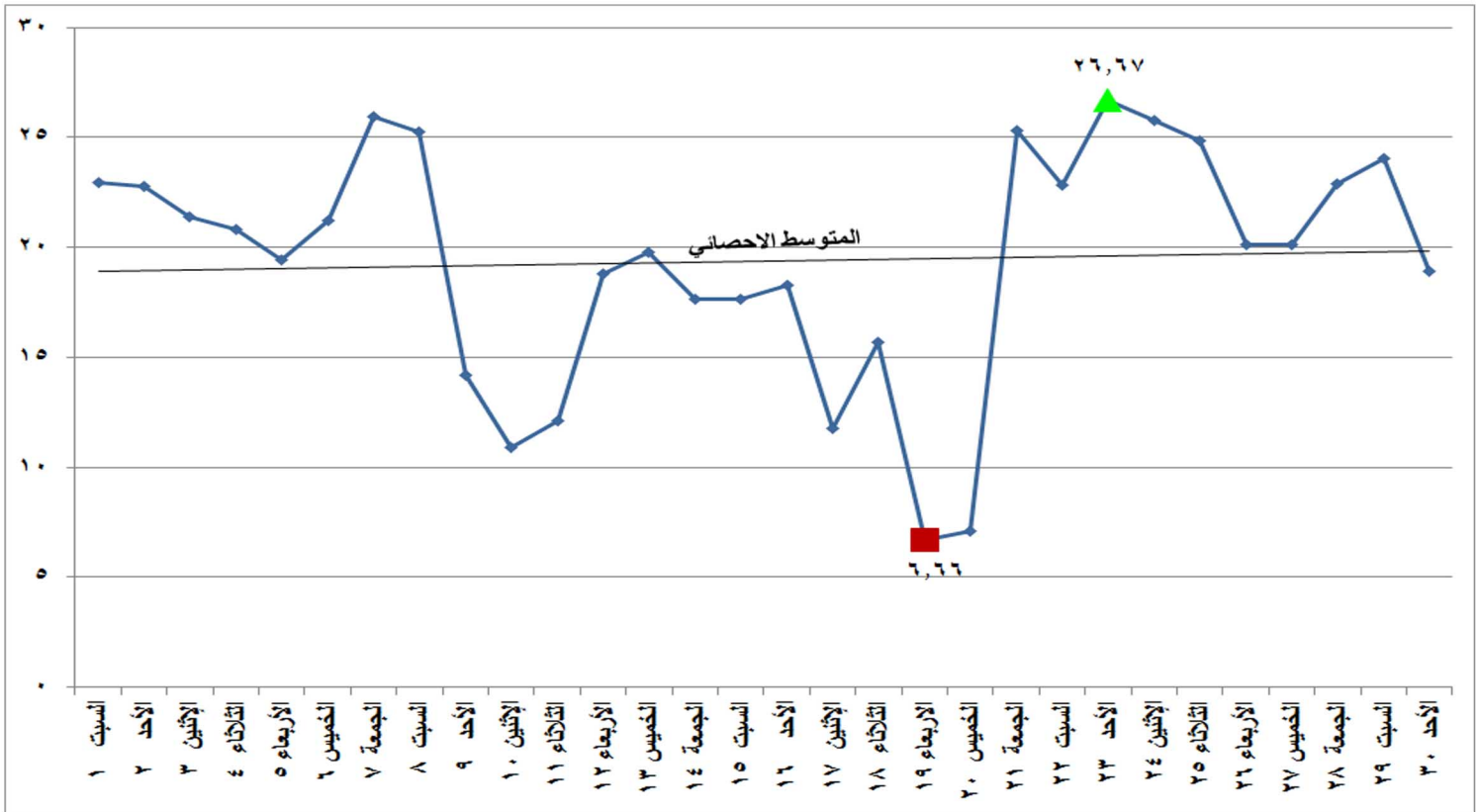
شكل (٢٥) الطاقة الكهربائية المنتجة من الرياح والشمس خلال شهر يونيو ٢٠١٩
