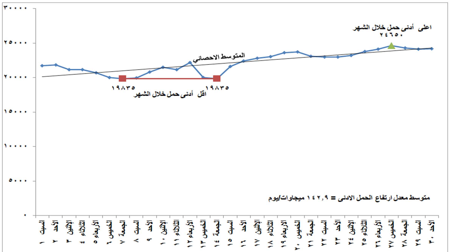
شكل (٢) تطور الحمل الادنى اليومي خلال شهر يونيو ٢٠١٩
