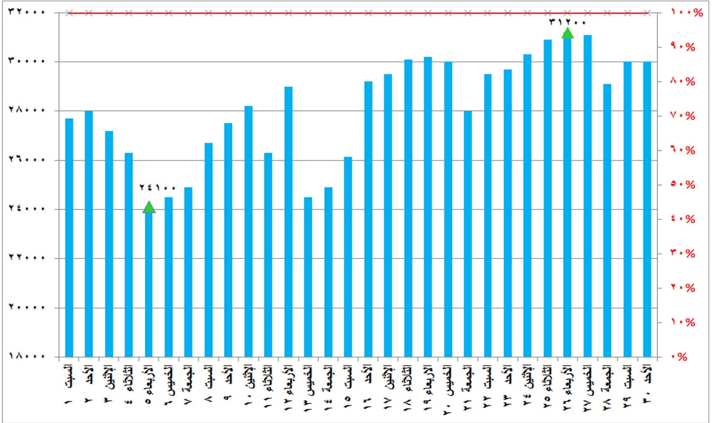
شكل (٥) قدرات الانتاج المتاحة ونسبتها للحمل الاقصى خلال شهر يونيو ٢٠١٩
