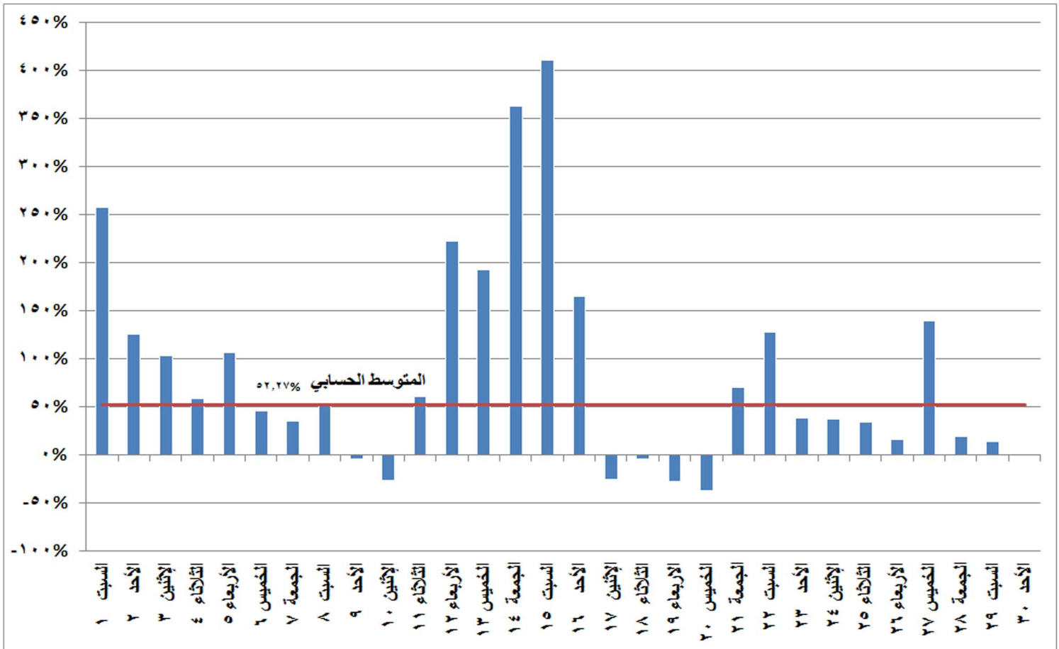
شكل (٢٦) نسب التغير في استخدام الرياح والشمس في إنتاج الطاقة الكهربائية خلال شهر يونيو ٢٠١٩ مقارنة بالشهر المماثل من العام السابق
