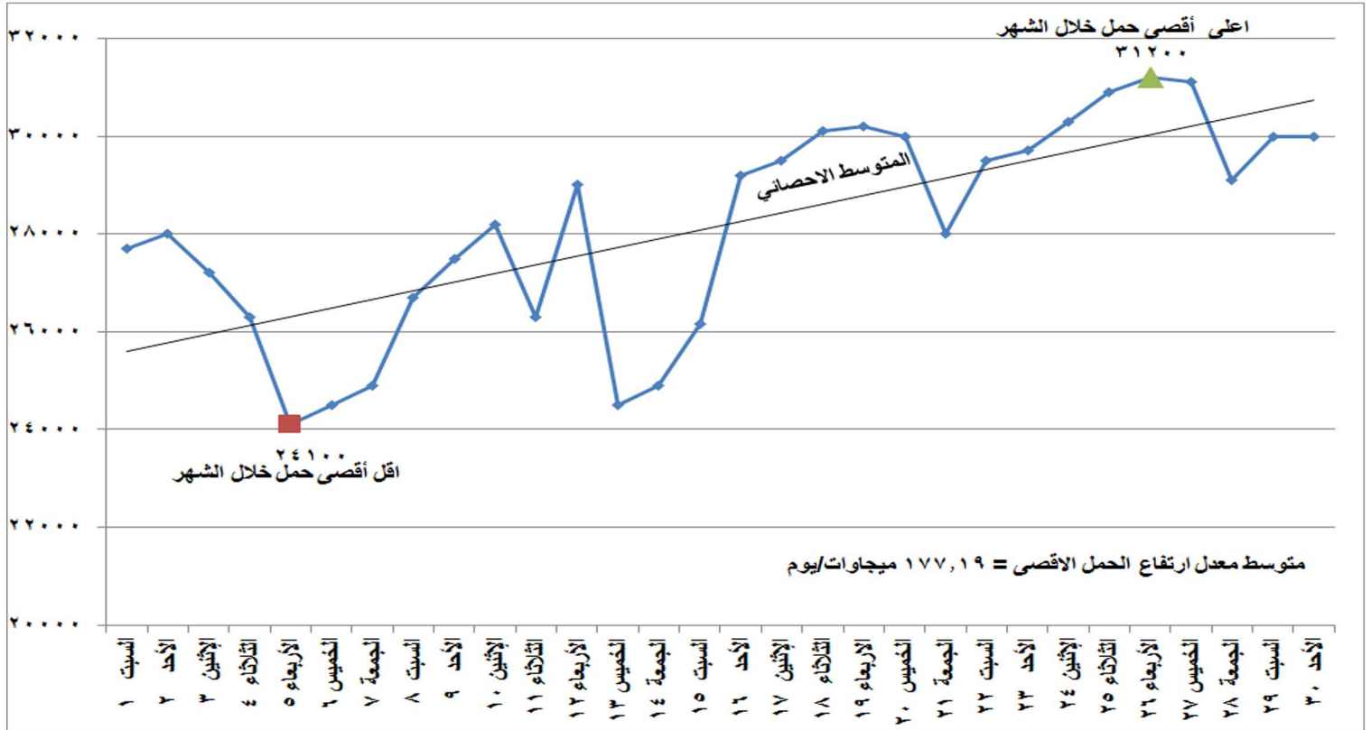
شكل (١) تطور الحمل الاقصى اليومي خلال شهر يونيو ٢٠١٩
