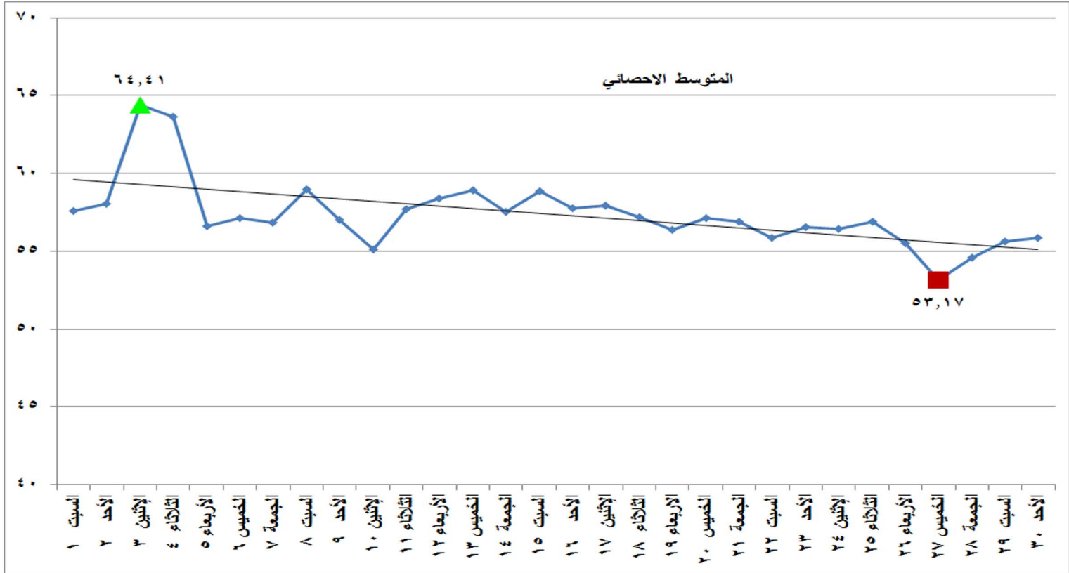
شكل (٢٣) الطاقة الكهربائية المنتجة من المصادر المائية خلال شهر يونيو ٢٠١٩
