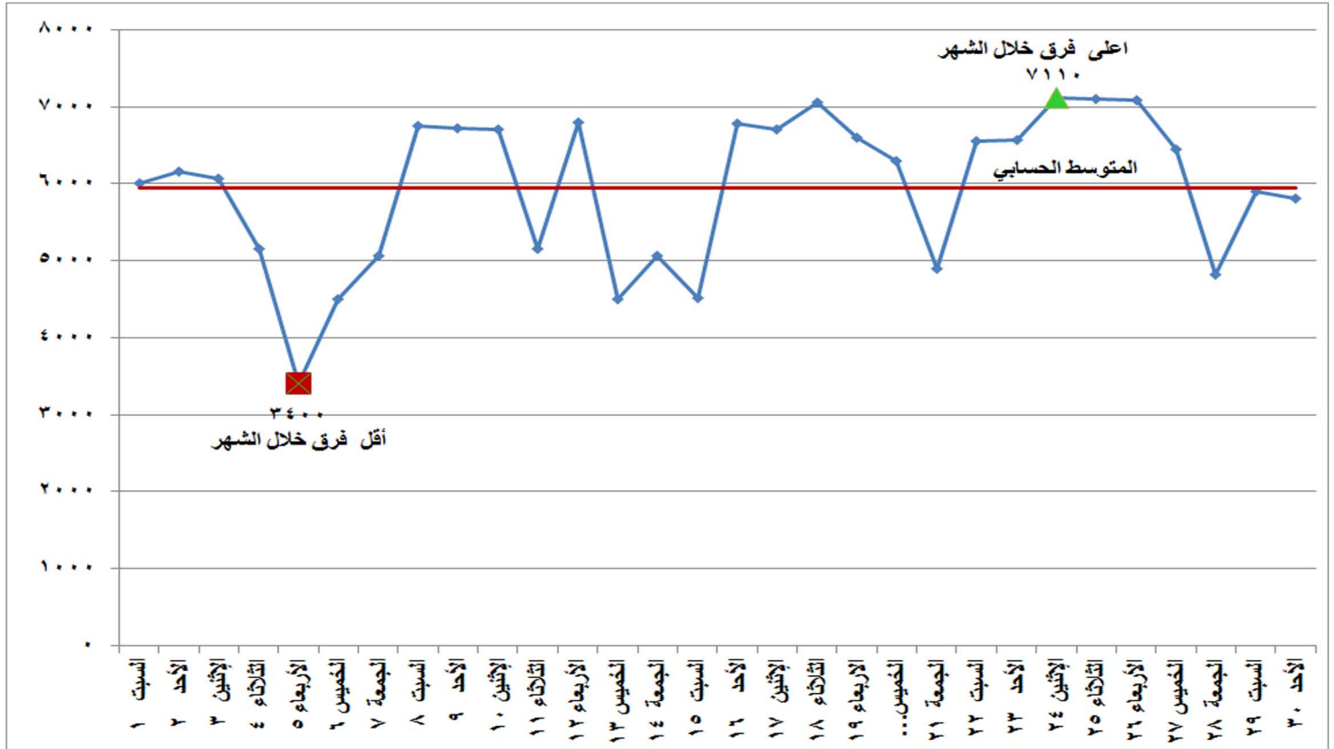
شكل (٣) الفرق بين أقصى وأدنى حمل خلال شهر يونيو ٢٠١٩
