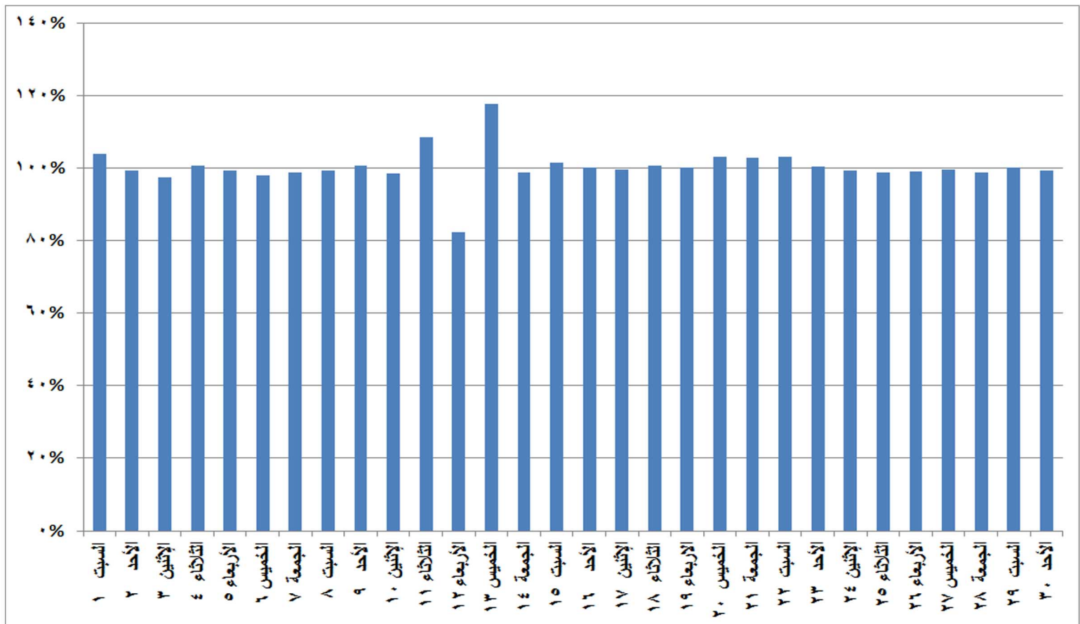
شكل (٢٨) نسب الفائض للحمل الاقصى المسجل يوميا خلال شهر يونيو ٢٠١٩
